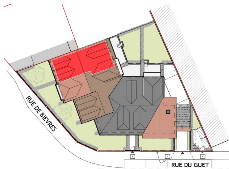
Plan masse
